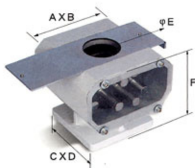
Magnet box + Magnet base 磁鐵盒+磁鐵座
