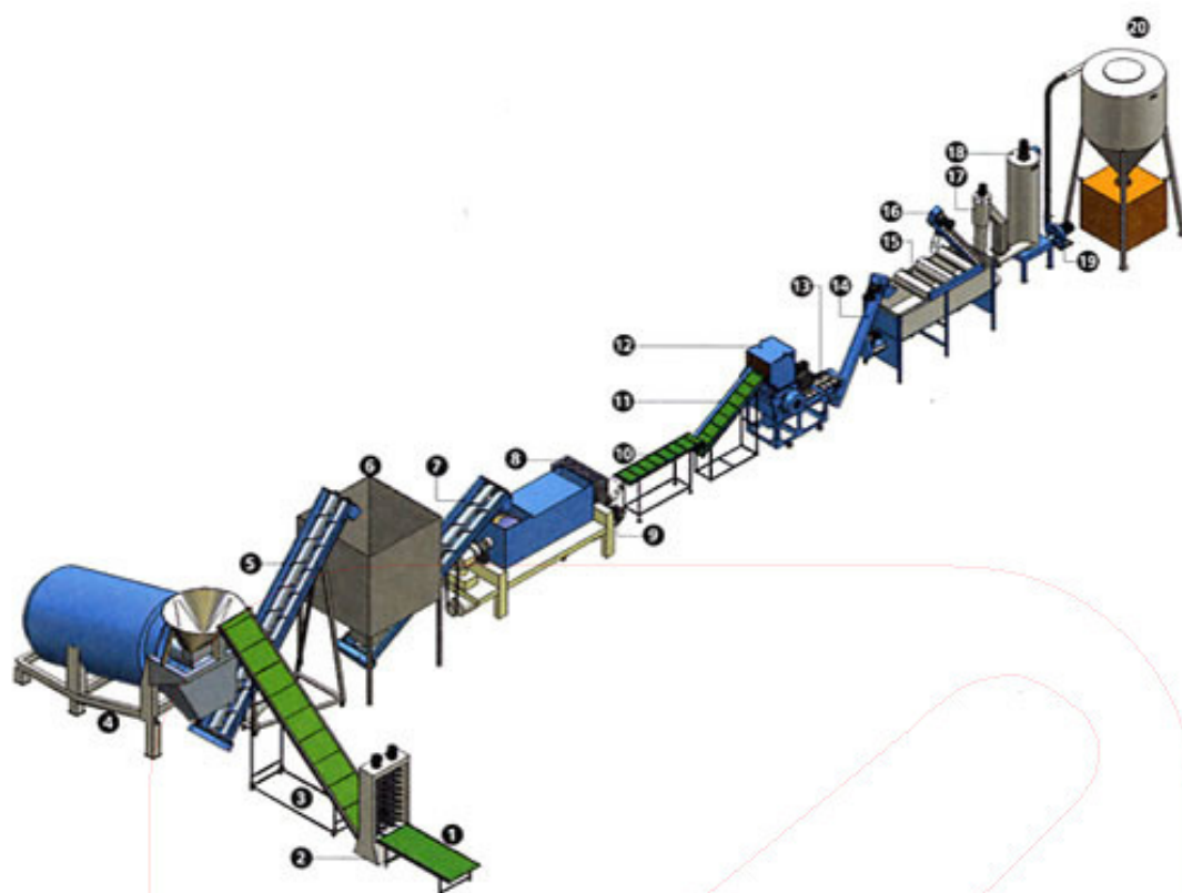
濕式粉碎PET瓶回收系統圖
