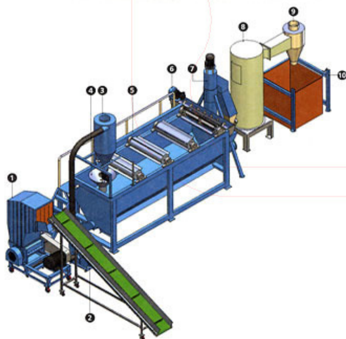
乾式粉碎PET瓶回收系統圖
