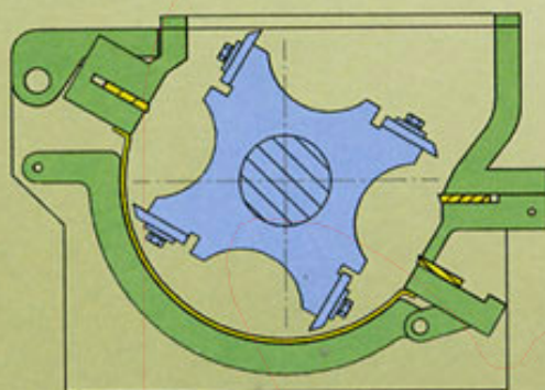
cutting chamber 刀室示意圖
