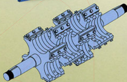
rotor 刀輪示意圖
